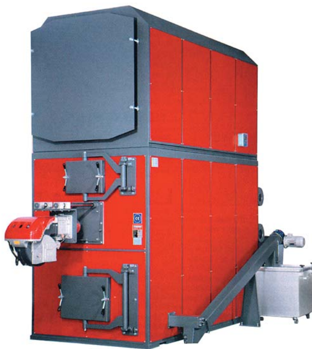
Model kotlovnice Uniconfort za vlažnu biomasu
