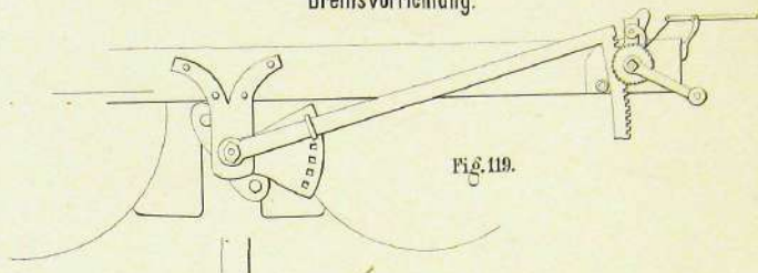
Bremsvorrichtung.
