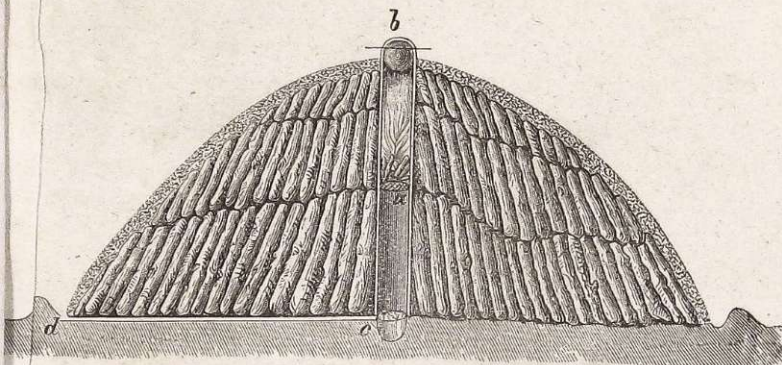
a Der Koff. b Die Kugel zum verschließen. cd Der Zugcanal.
