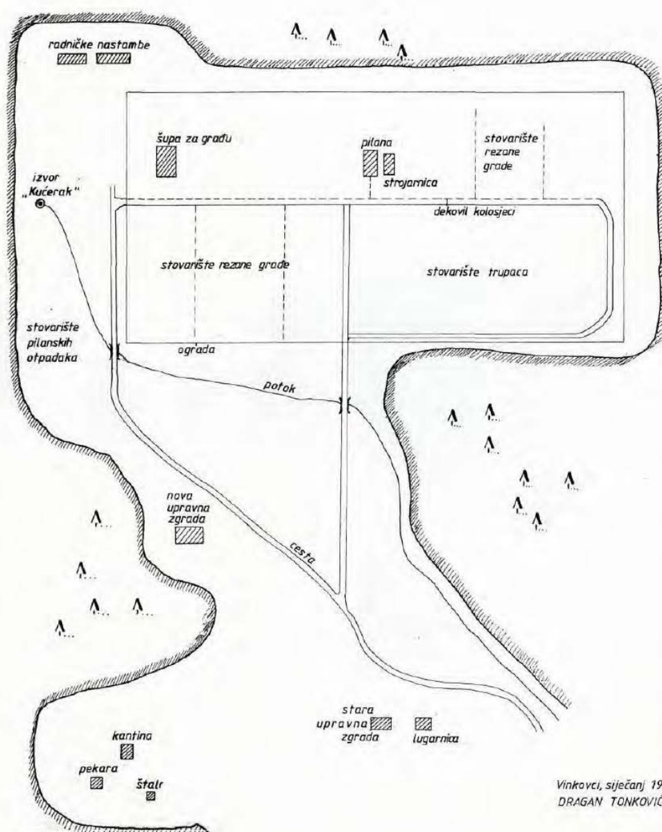
skica PILANSKIH POSTROJENJA I ZGRADA NA ŠTIROVAČI PREMA STANJU 1940. god.
